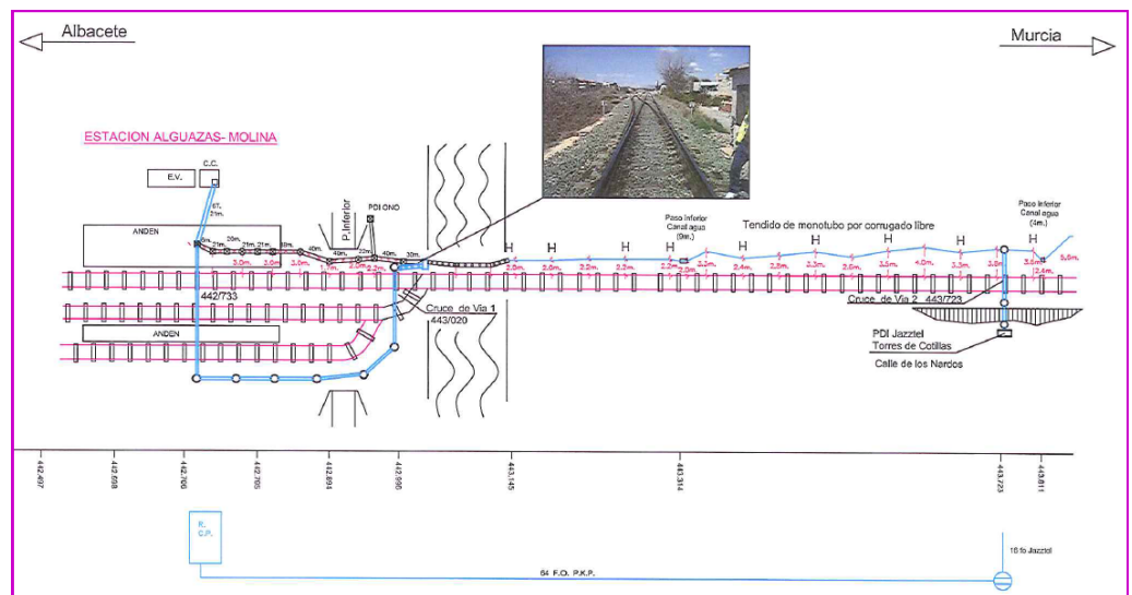
Ejemplo de un plano inicial del Proyecto de enlaces de Jazztel en las Torres de Cotillas
